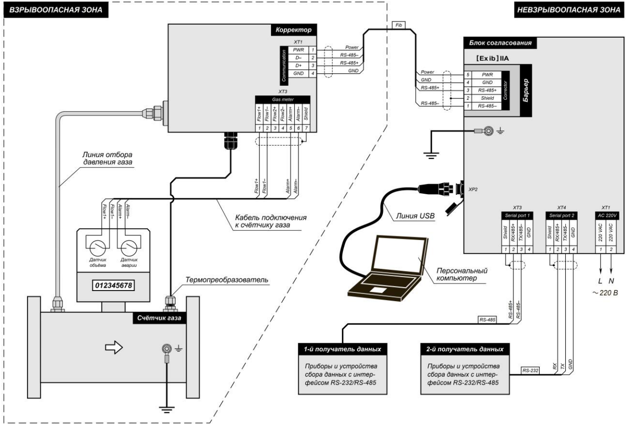
Рисунок В.9 Подключение корректора с применением блока согласования «Суперфлоу 23 БС»
