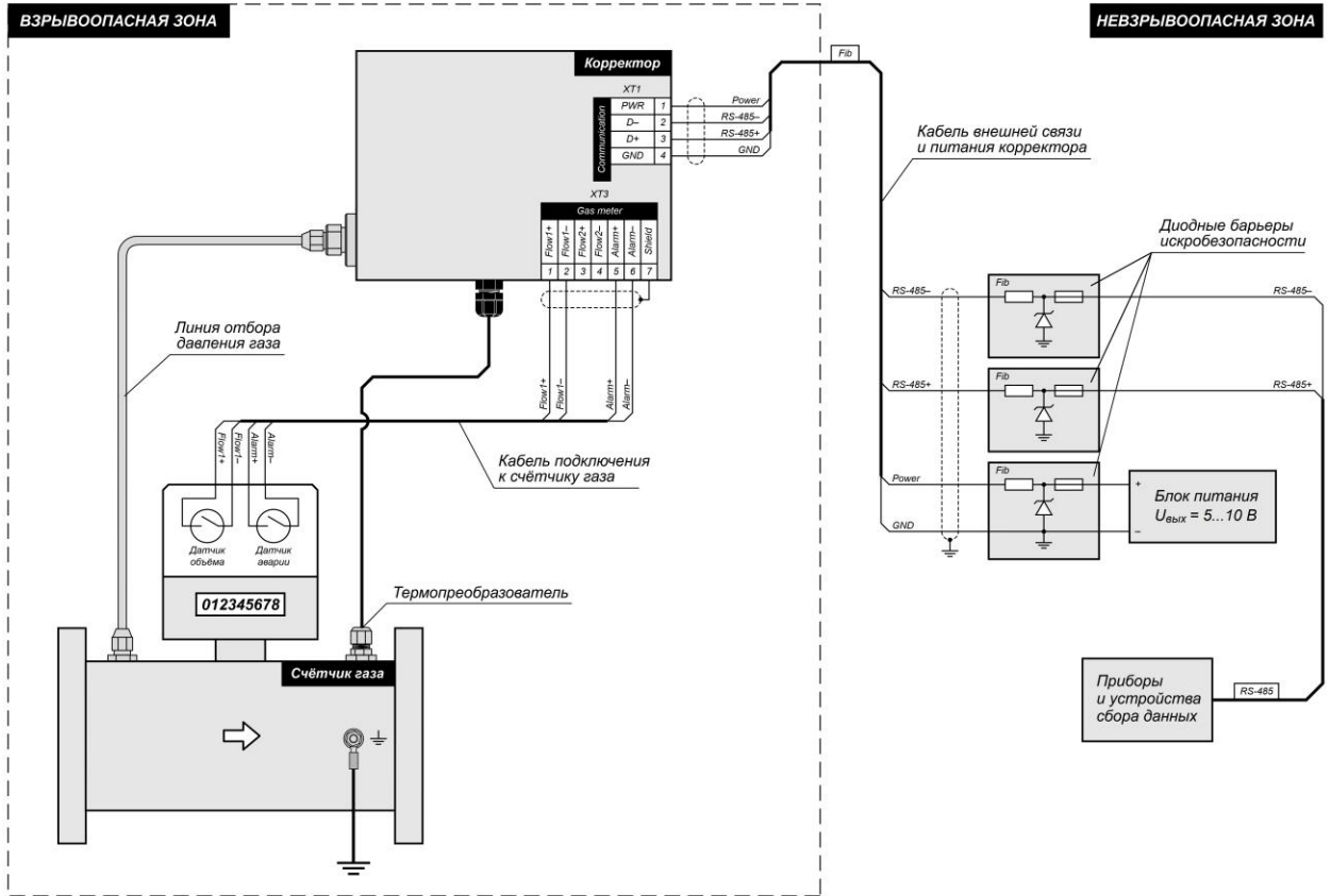
Рисунок В.8 Обобщённая схема подключения корректора к внешнему оборудованию
