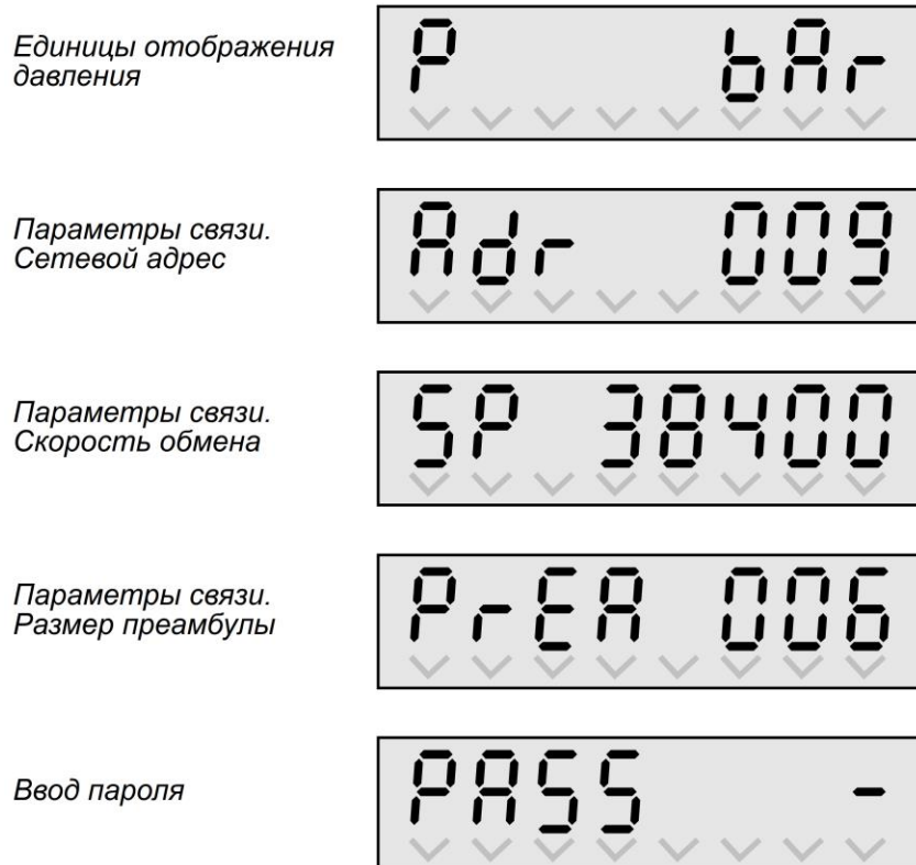
Рисунок 46 Параметры рабочего режима из меню «SEtInGS»
