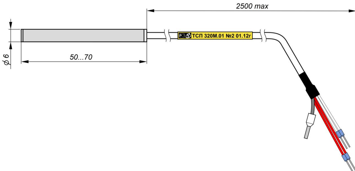
Рисунок Б.2 Термопреобразователь
