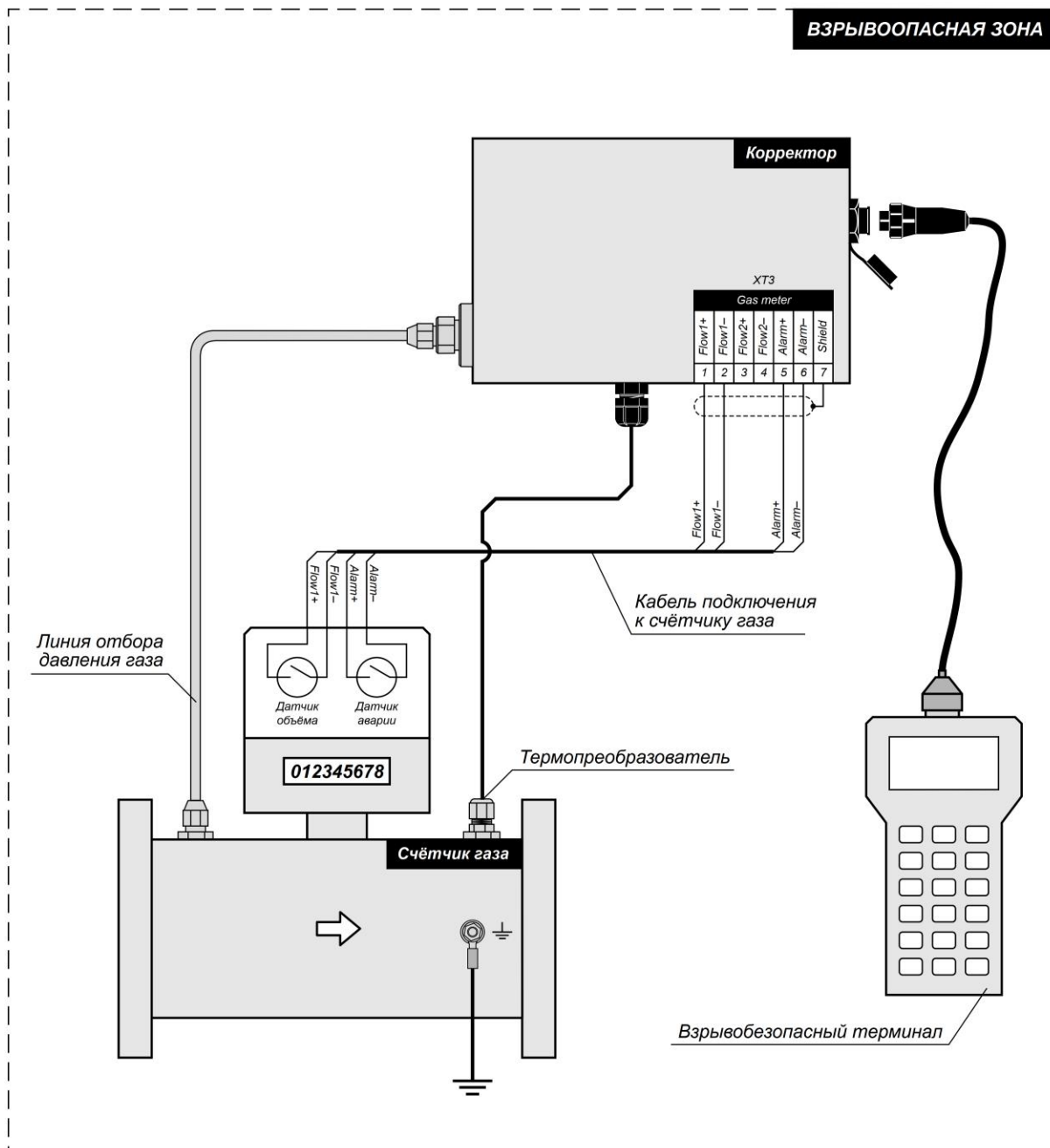
Рисунок В.6 Считывание архивных данных во взрывоопасной зоне с использованием взрывобезопасного терминала
