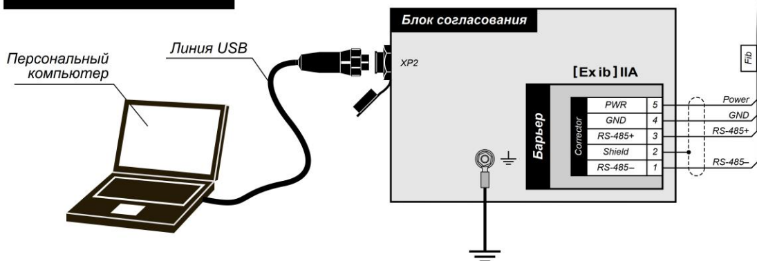
Рисунок В.7 Считывание архивных данных во взрывоопасной зоне с использованием компьютера и блока согласования «Суперфлоу 23 БС»
