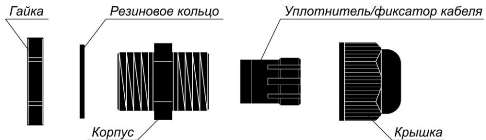
Рисунок 9 Конструкция кабельного ввода
