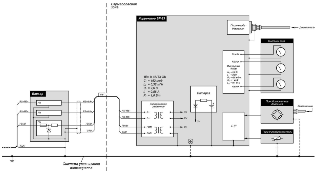
Рисунок 4 Обобщённая схема обеспечения взрывозащищённости
