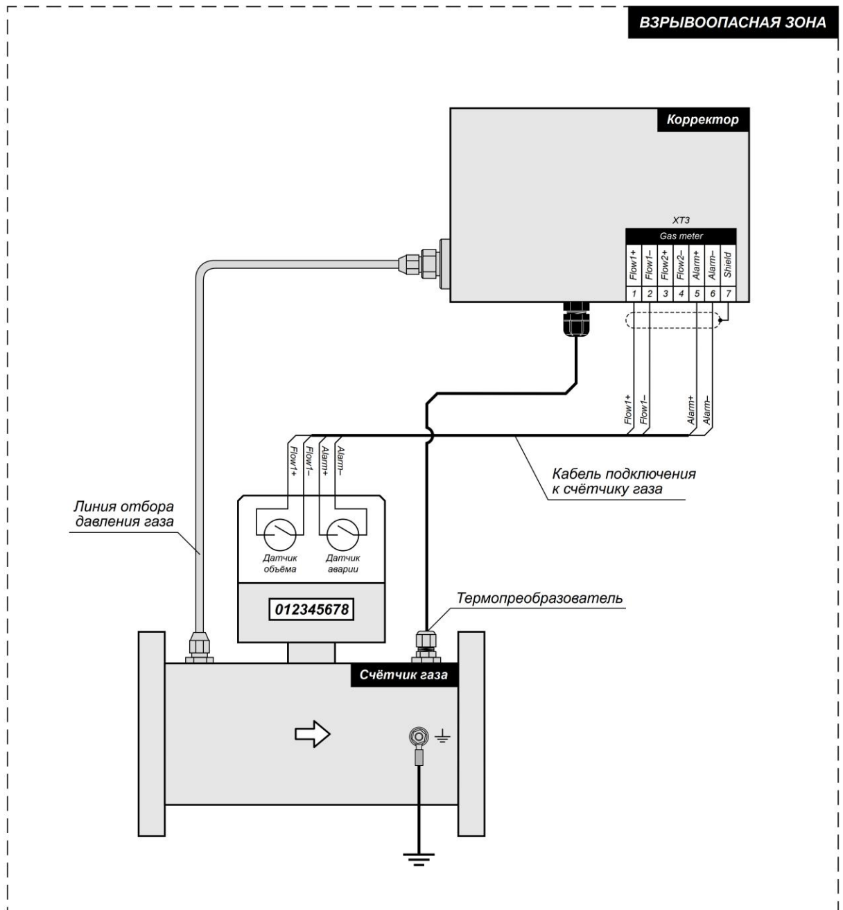
Рисунок В.1 Простейший вариант подключения корректора
