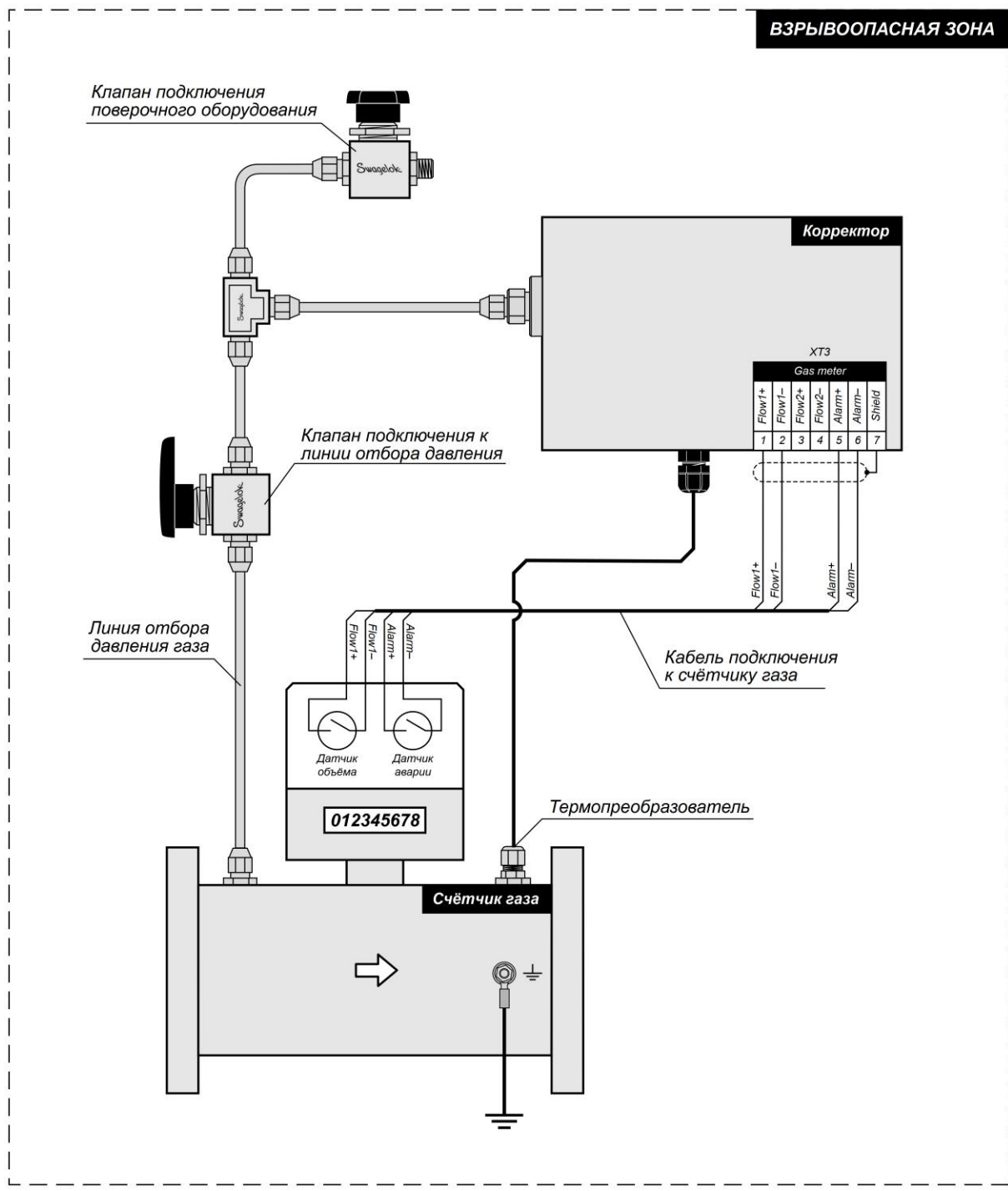
Рисунок В.4 Установка клапанов для линии подключения поверочного оборудования
