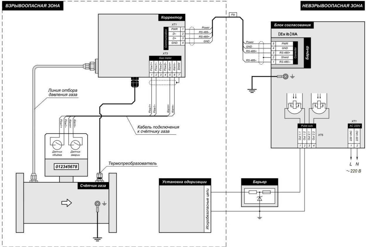
Рисунок В.11 Вариант использования корректора для управления установкой одоризации с искробезопасными цепями
