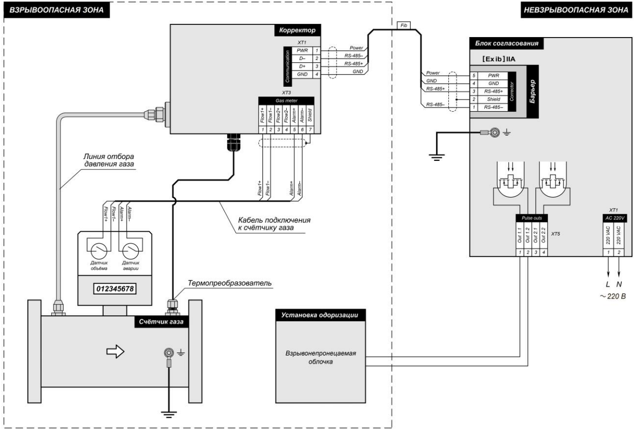
Рисунок В.10 Вариант использования корректора для управления установкой одоризации во взрывонепроницаемой оболочке
