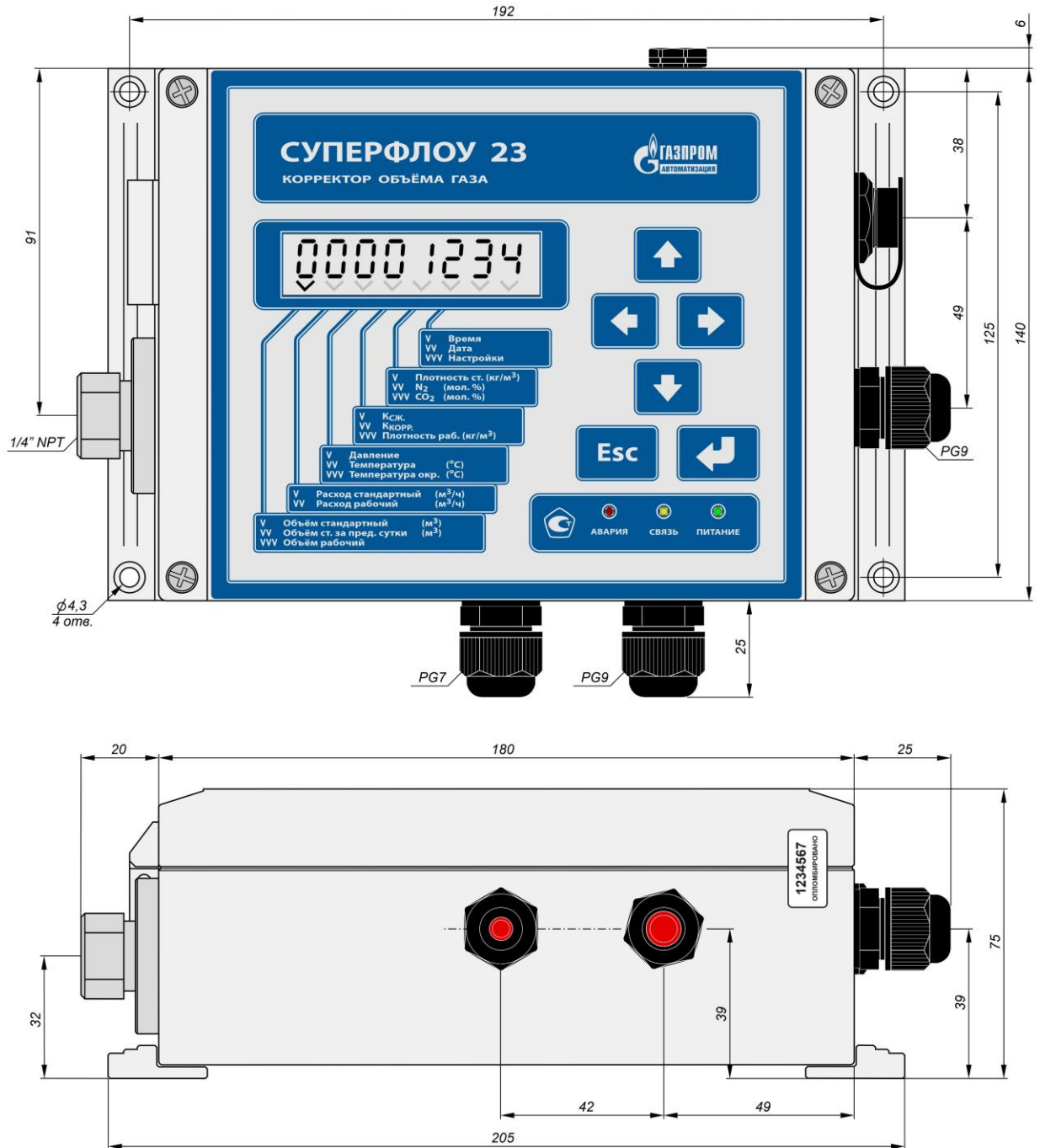
Рисунок Б.1 Корректор объёма газа
