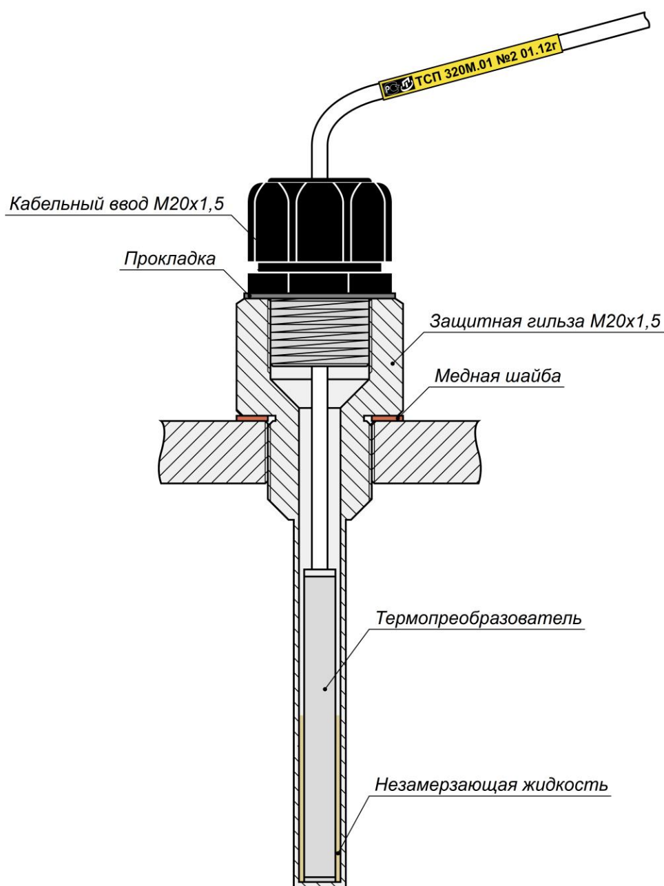
Рисунок 8 Монтаж термопреобразователя
