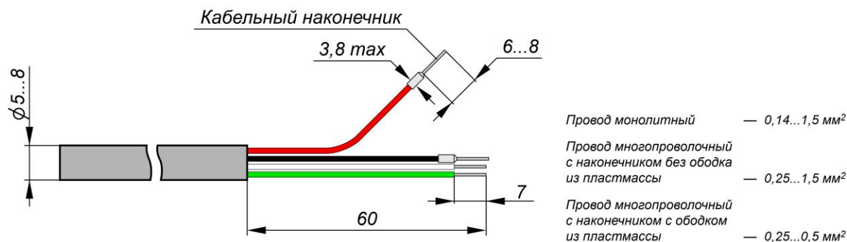
Рисунок 10 Подготовка кабеля
