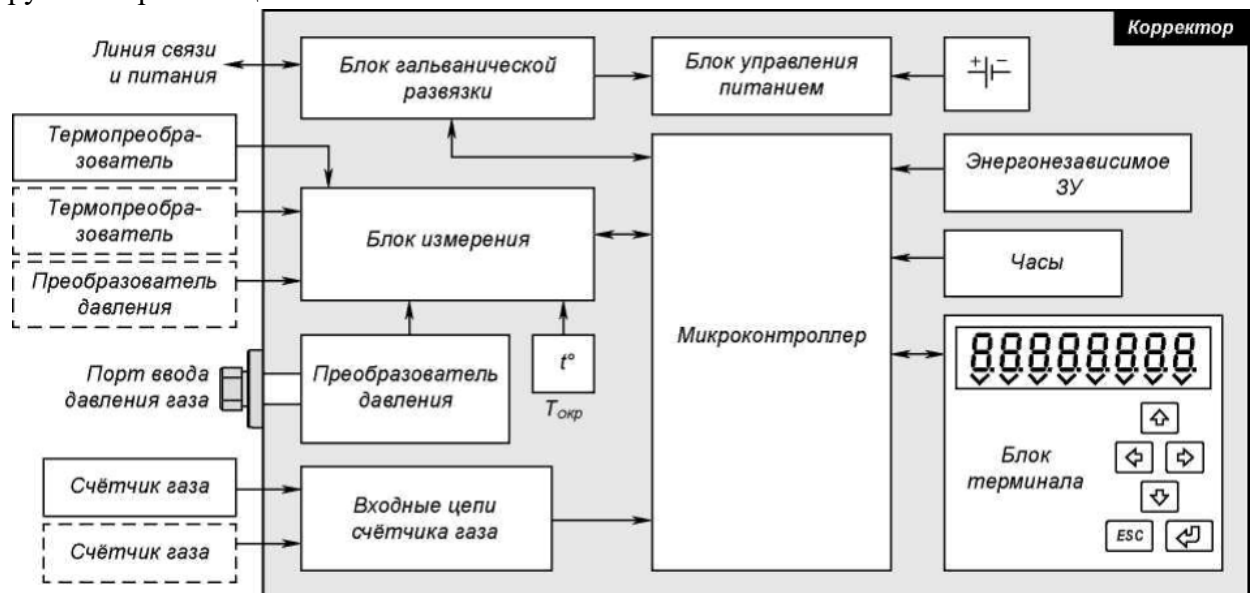
Рисунок 2 Структурная схема корректора
