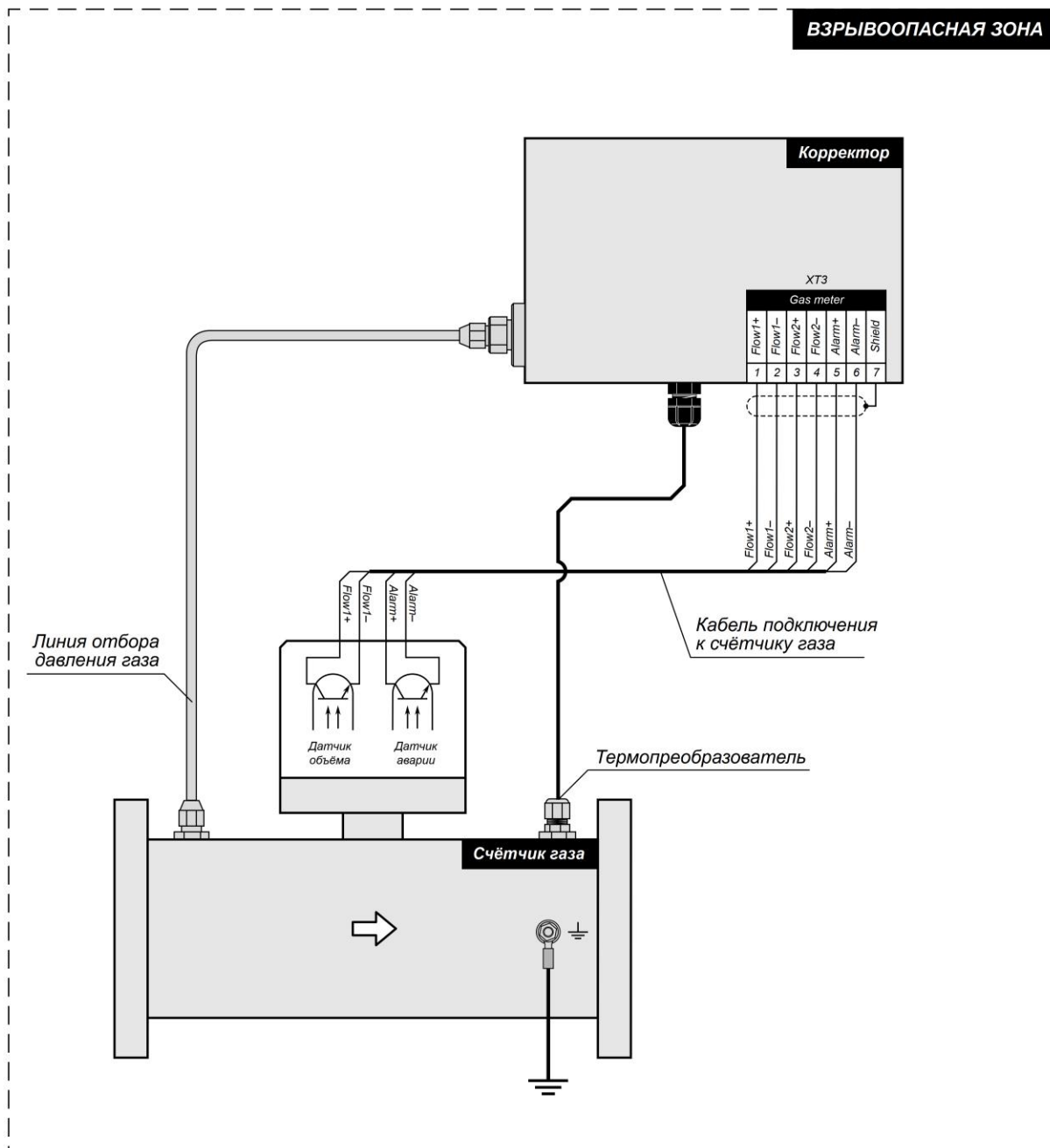
Рисунок В.3 Подключение к счётчику газа с выходами на базе электронных ключей
