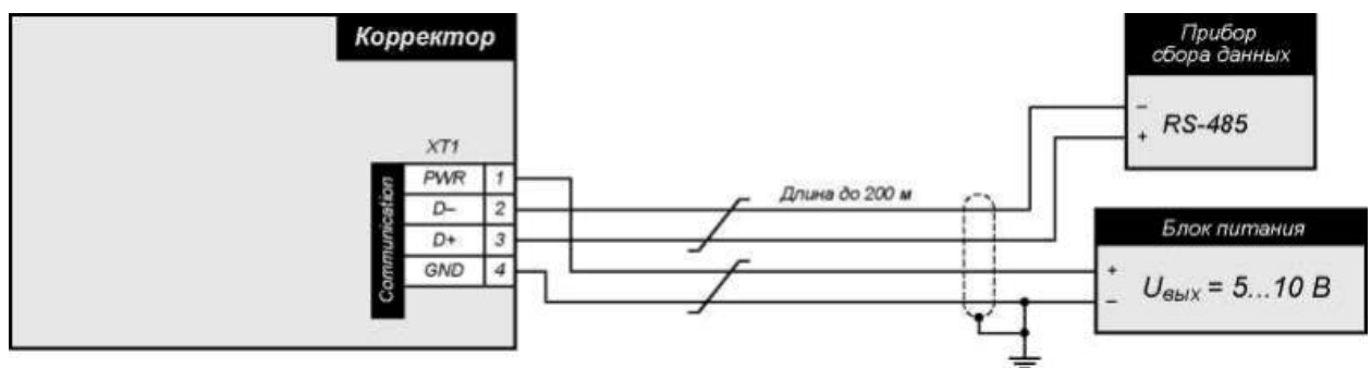
Рисунок 15 Схема подключения линии связи и питания
