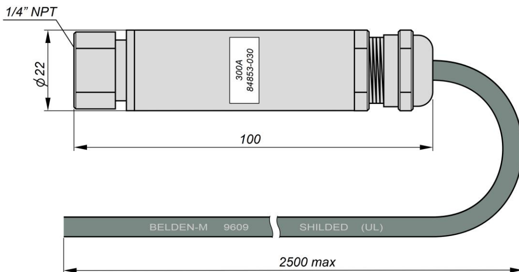
Рисунок Б.3 Выносной преобразователь давления
