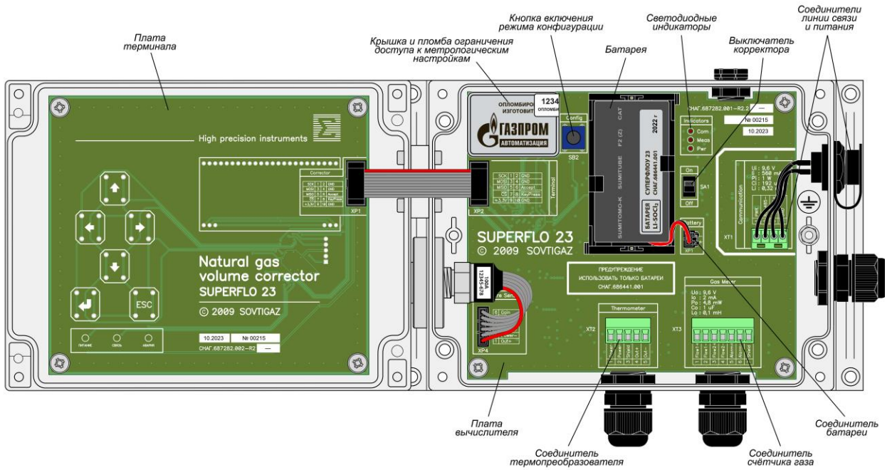
Рисунок 3 Вид корректора с открытой крышкой
