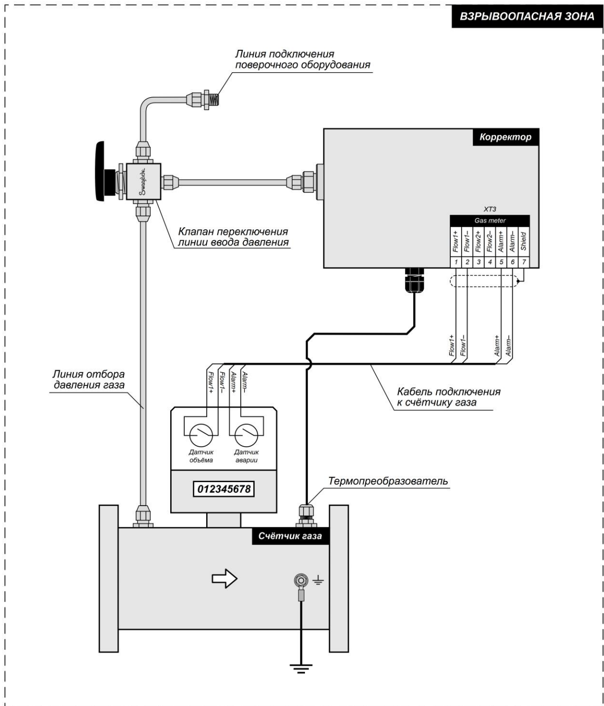
Рисунок В.5 Подключение с использованием 3-ходового переключающего клапана
