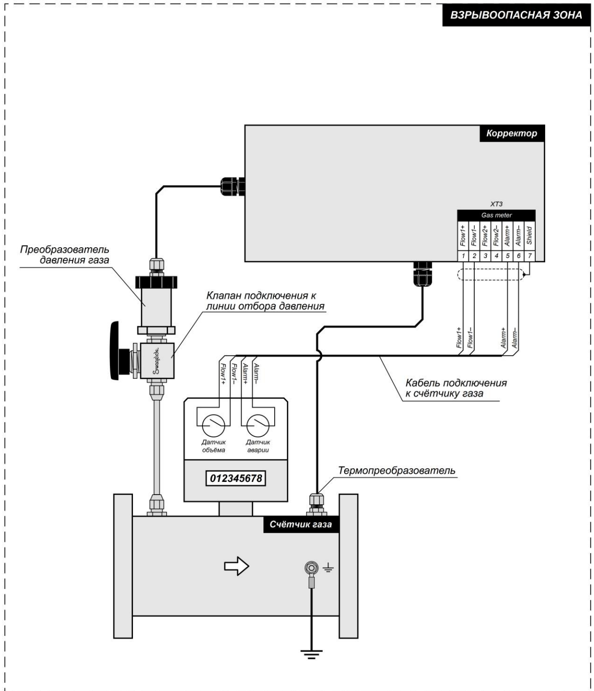
Рисунок В.14 Установка выносного преобразователя давления
